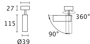
Ø66.8 Z232CC Mini Track canope
