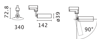
Z232CZ Mini Track riel
